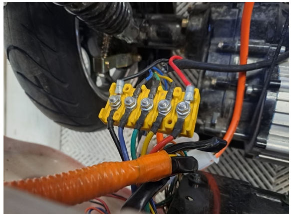
Irrota kytkentärimaan kytkettyjen johtimien kiinnitysmutterit. (hylsy 8 mm).
