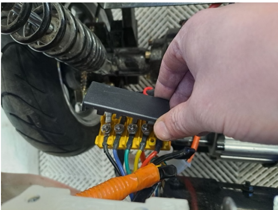
Avaa päävirran kytkentäriman kansi
